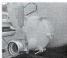
Tampa de inspeção de 550 mm e pistão pneumático de abertura do registro
