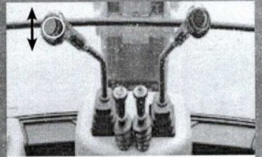
Acionamento de escavação conforme ISO.
