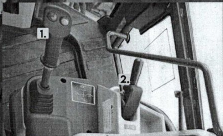
1. Caçamba com nivelamento automático durante o processo de levantamento do braço, com variação de até 1,5° na caçamba.
